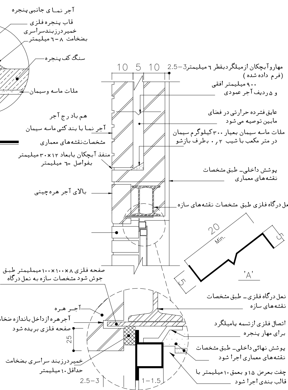
جزئیات دیوار دو جداره
