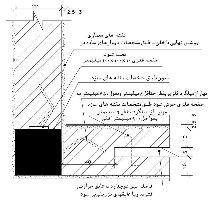
جزئیات اتصال ستون به دیوار
