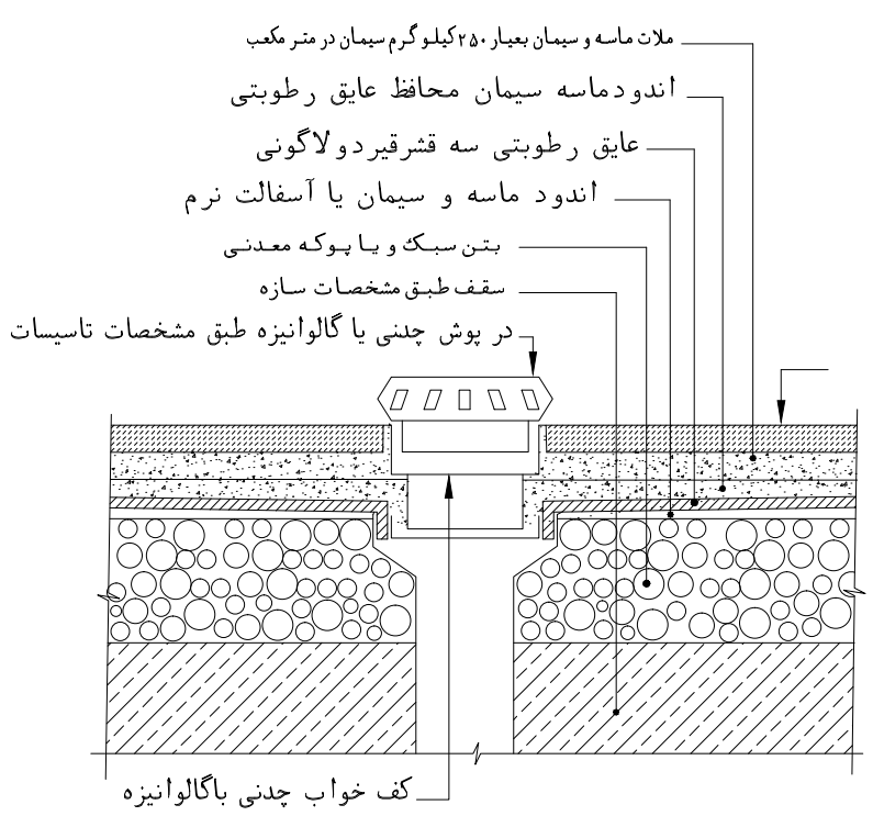
جزئیات کف سازی و آبروی بام
