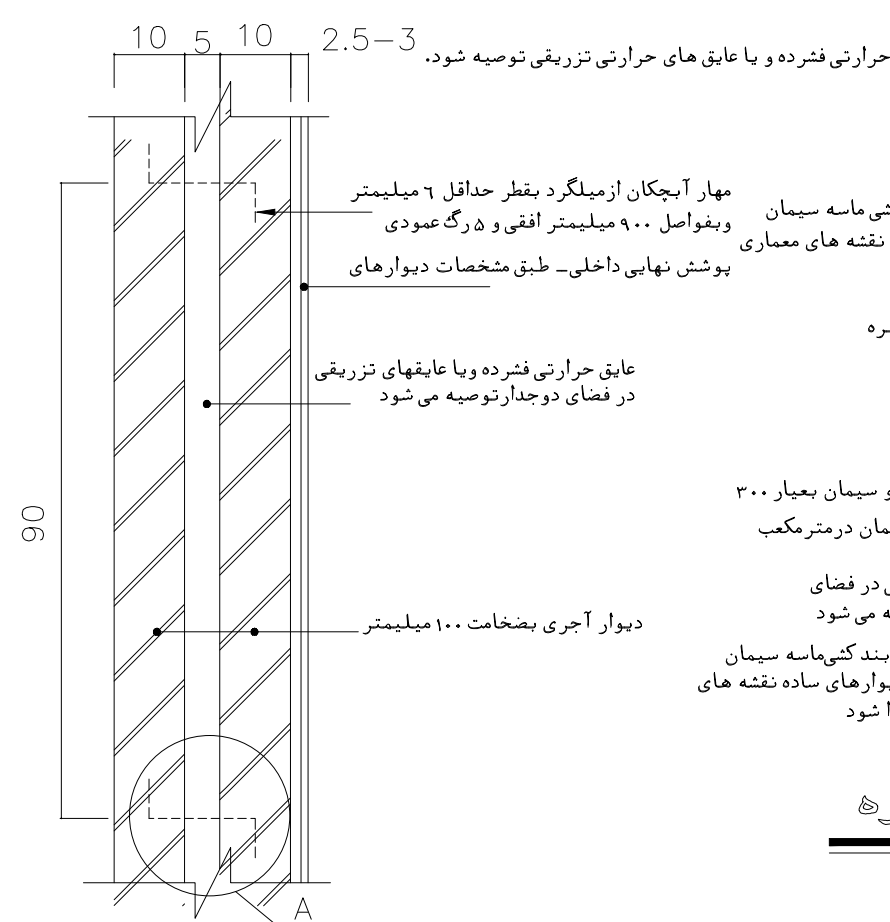
جزئیات دیوار دو جداره
