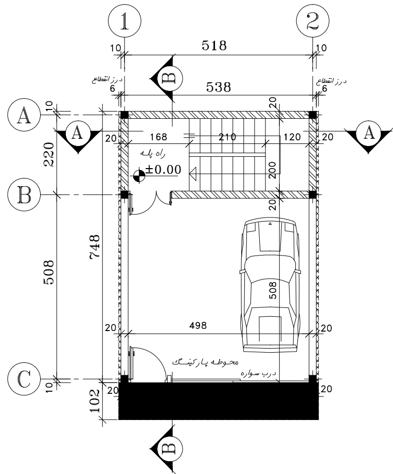
پلان اندازه گذار و طبقه مهمکف
