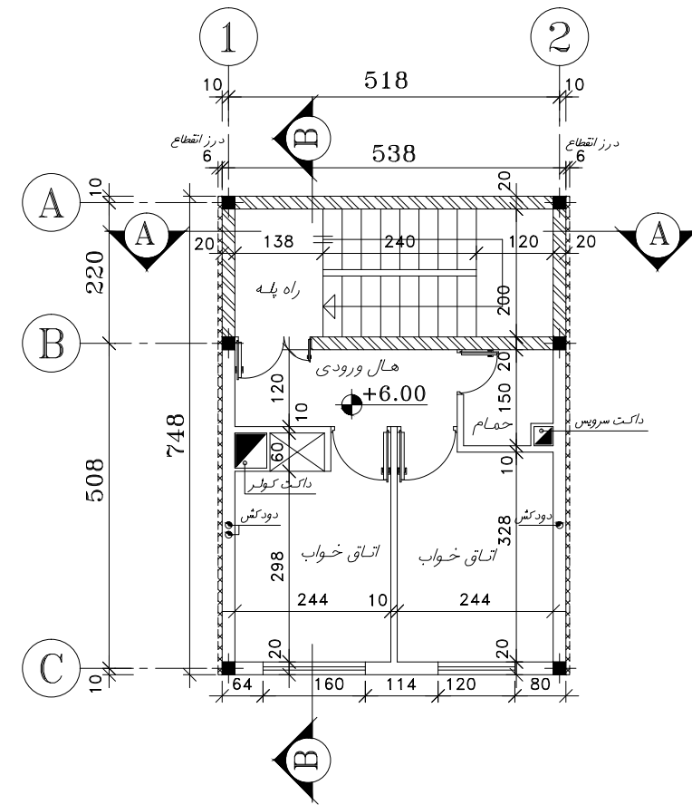
پلان اندازه گذار و طبقه دو و بالکس
