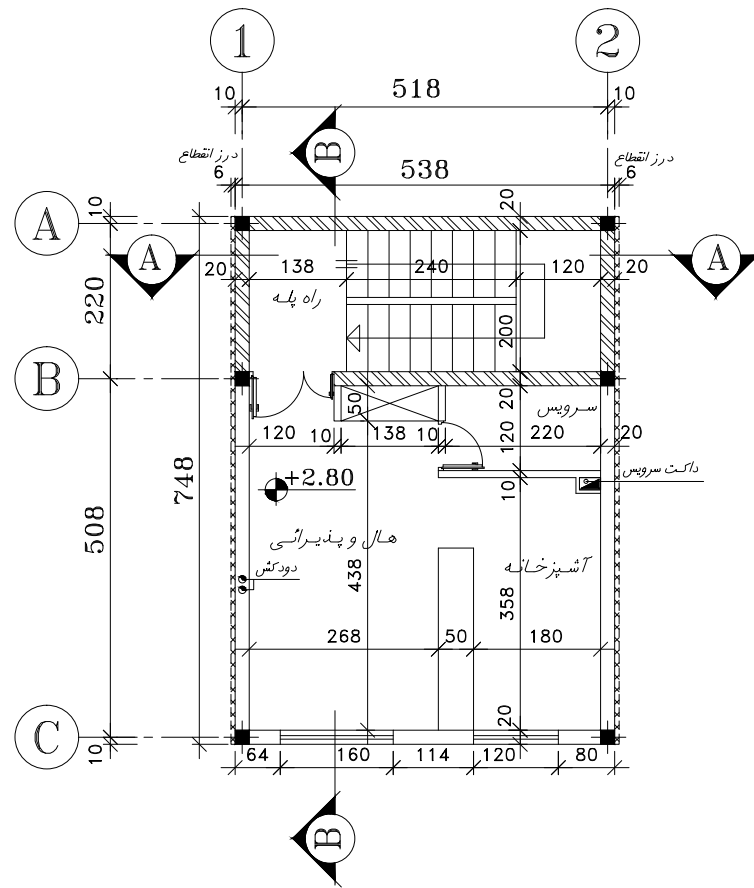
پلان اندازه گذار و طبقه اول
