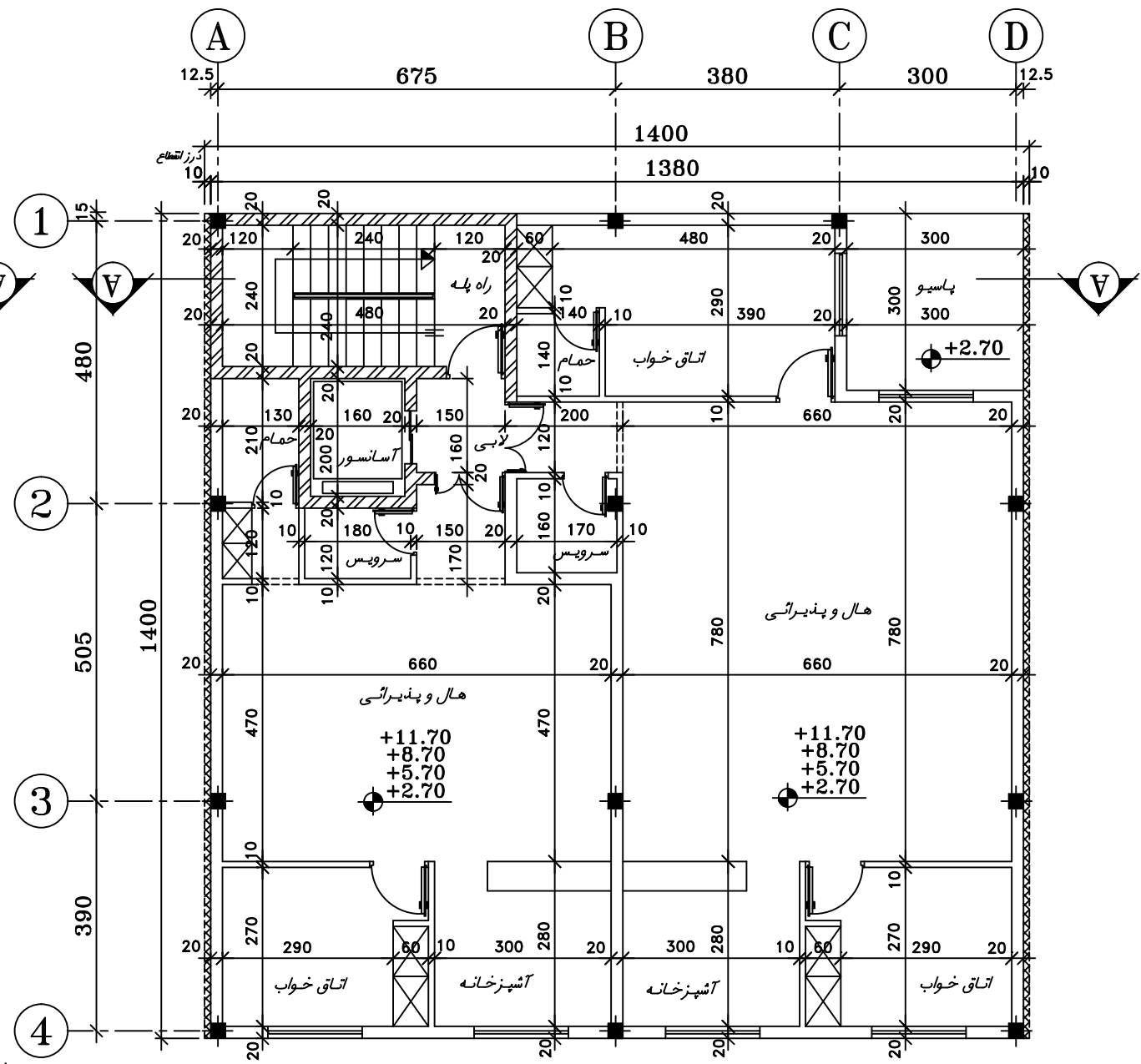
پلان اندازه گذاری طبقه اول ای چهارم SC.1:100 مسکونی دو واحدی
