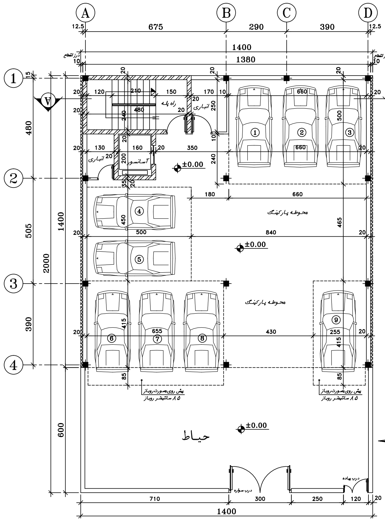
پلان اندازه گذاری طبقه همکف SC.1:100
